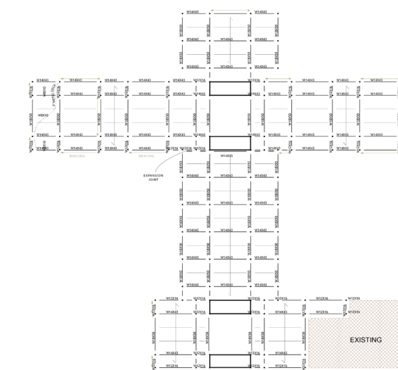
Primer Nivel First Level
