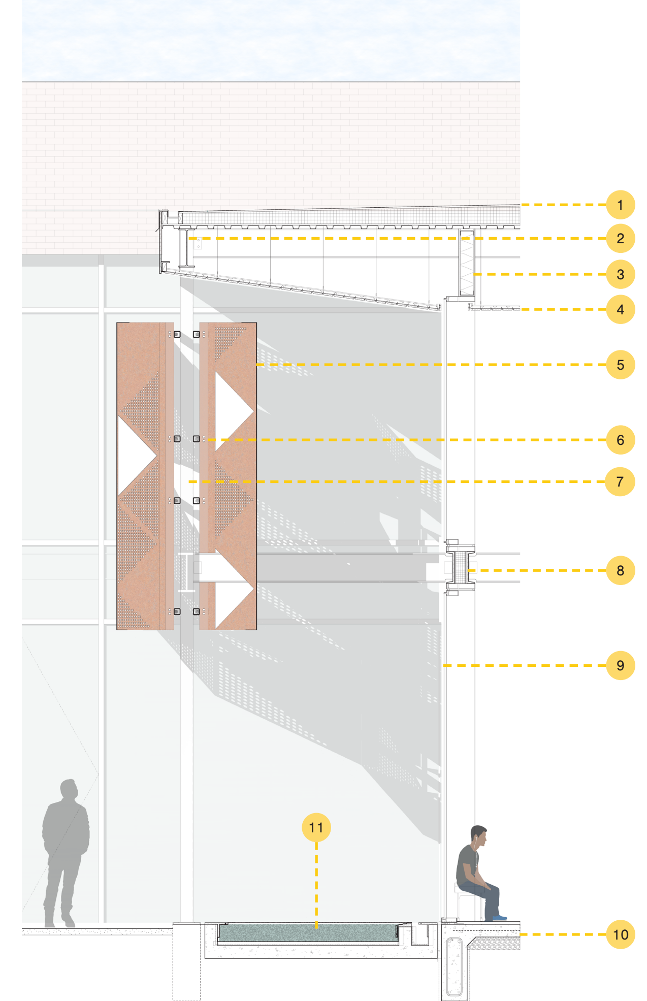
Corte Detallado Section Detail
