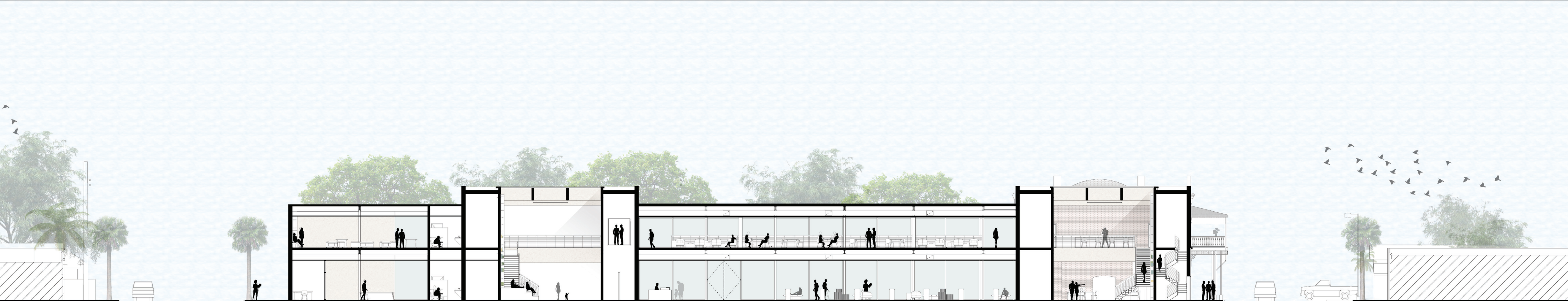
Corte Longitudinal Longitudinal Section
