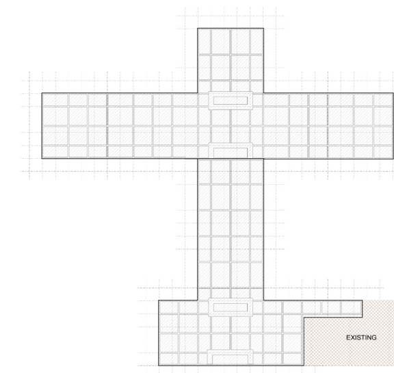
Planta De Cimentación Foundation
